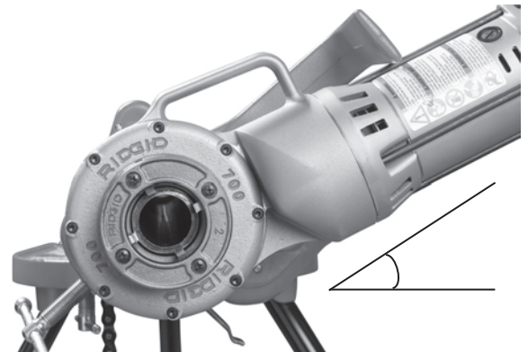
Figura 6 – Brazo de soporte con el accionamiento motorizado 700 colocado ligeramente encima de la línea horizontal
