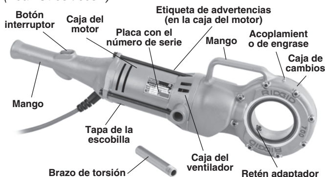
Figura 1 – Accionamiento motorizado Modelo 700
